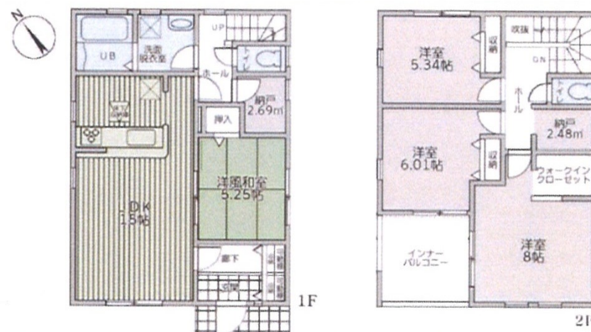
【間取り図】
